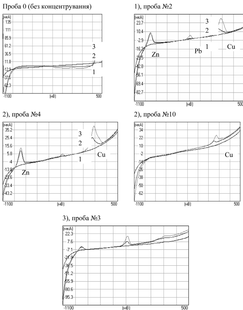
Рис.1 Приклади кривих інверсійно-вольтамперометричного визначення іонів цинку, плюмбуму та купруму в різних порціях елюатів, отриманих шляхом кислотного відмивання адсорбційного патрону PuCOONa-CX після пропускання через нього 1000 мл води з бювету: 1) пр. Бажана; 2) пр. Григоренка; 3) вул. Драгоманова ( V=10 мл, S=100 ): 1) бідистилат, 2) елюат, 3) елюат з добавкою.
