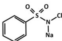
chloramine B
